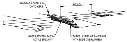
SANDBAG KERB INLET SEDIMENT TRAP N.T.S.
