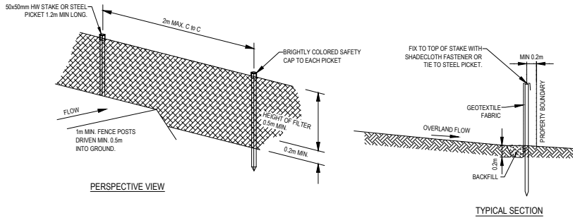
SEDIMENT FENCE DETAIL N.T.S.
